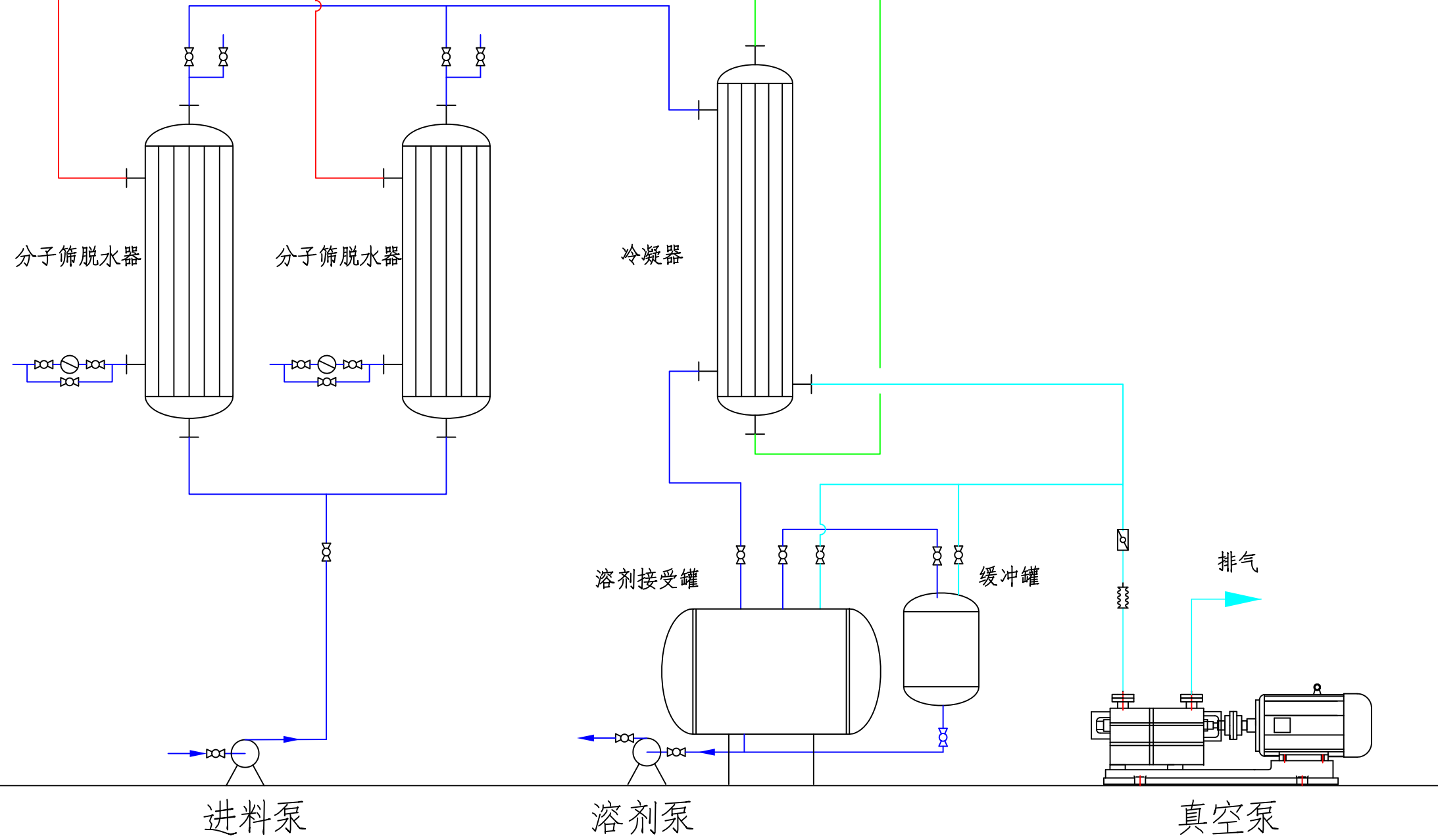
分子筛脱水工艺流程图
